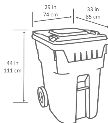
360 litre (95 gallon)
