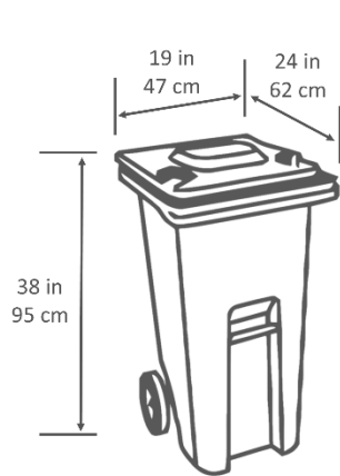
120 litre (35 gallon)
